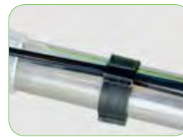
Waterslang code: 3.8023.107015 Bevestigingsclips om de waterslang aan de RVS zuigbuis te bevestigen code: 3.8023.107014
