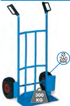
WP 415 Voetbasis: 470x270 mm Bestelnr. Prijs excl. BTW 770746 166 €
