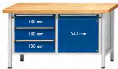
MOD. 106 V
