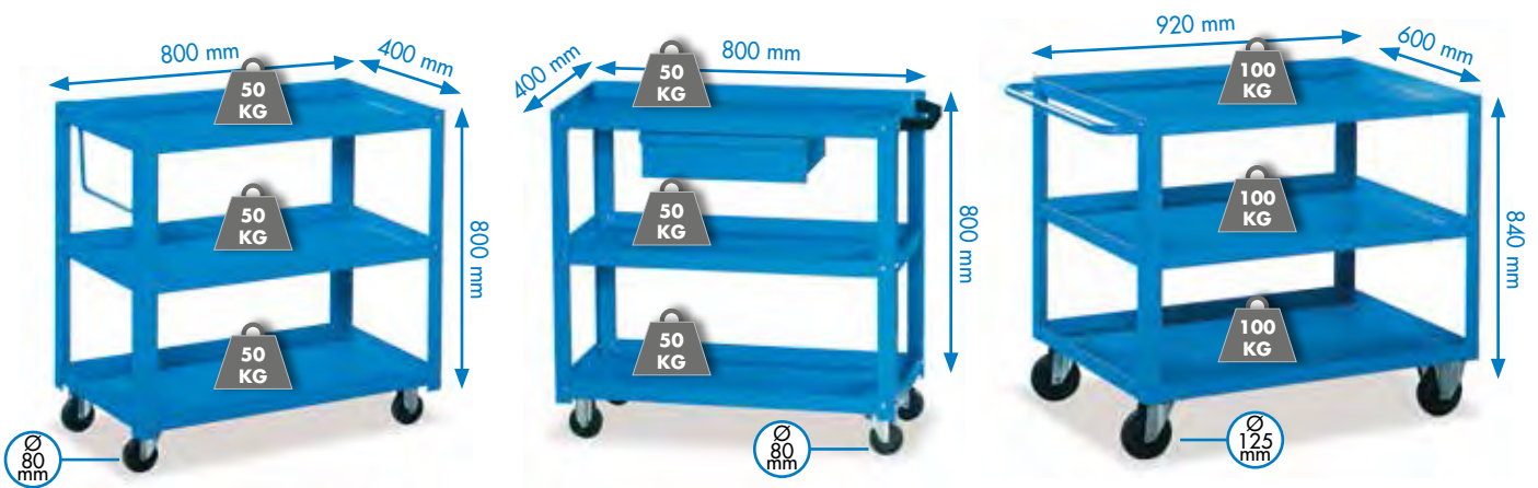
WP 402 Bestelnr. Prijs excl. BTW 770714 155 €
