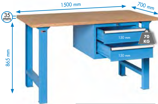
WP RX 150 01P Bestelnr. 776000 Prijs excl. BTW 569 €
