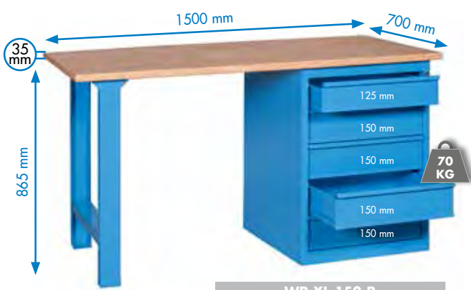
WP XL 150 P Bestelnr. 775968 Prijs excl. BTW 609 €
