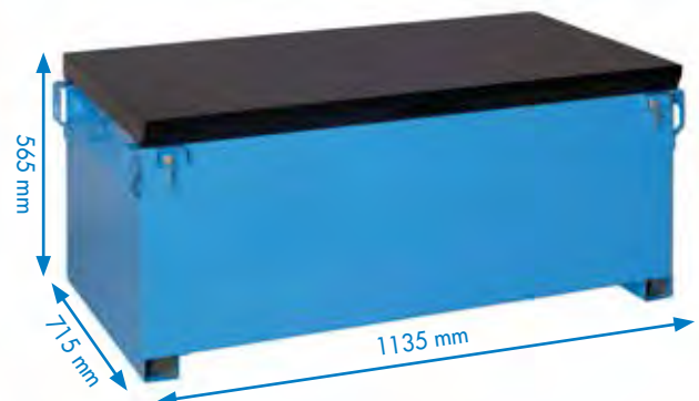
WP 227 Afsluitbaar: 2 sloten (links/rechts) Bestelnr. Prijs excl. BTW 770428 575 €
